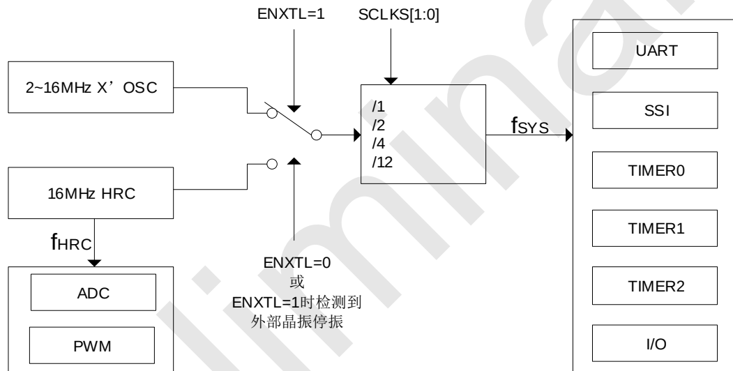
RD8G40x 内部时钟关系
