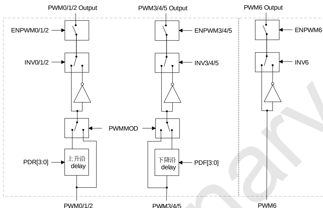
RD8G40x PWM 互补模式框图
