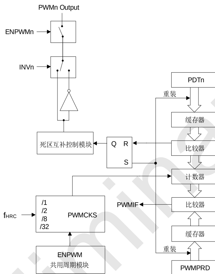
RD8G40x PWM 结构框图
