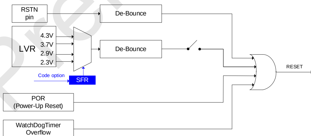
RD8G40x 复位电路图
