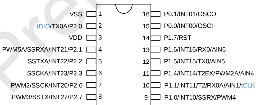
16PIN 管脚配置图
