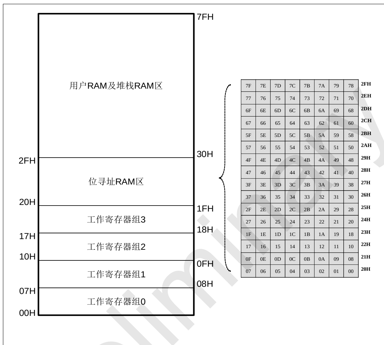
SRAM 结构图
