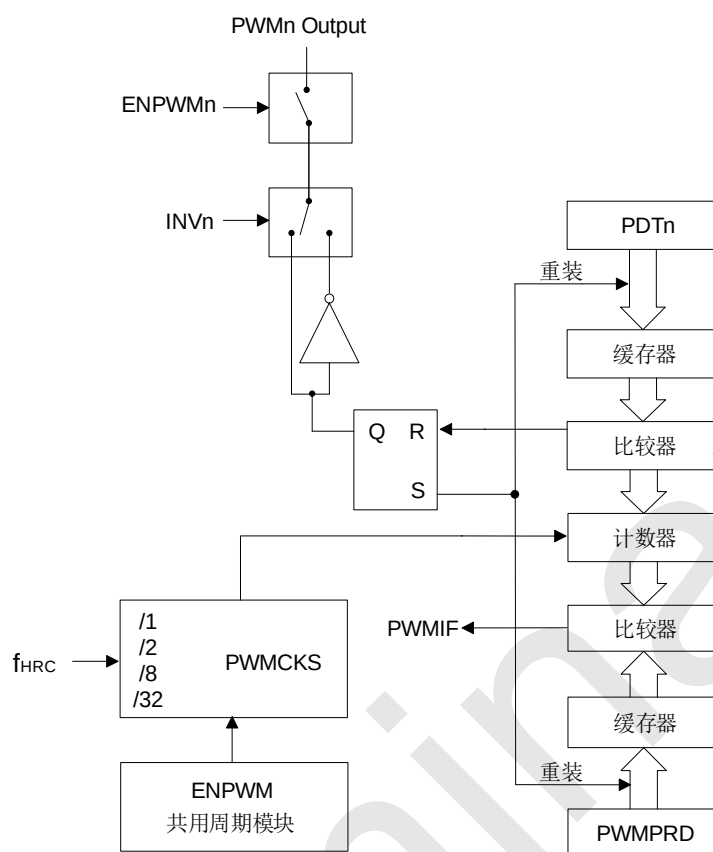
RD8G40x PWM 独立模式框图
