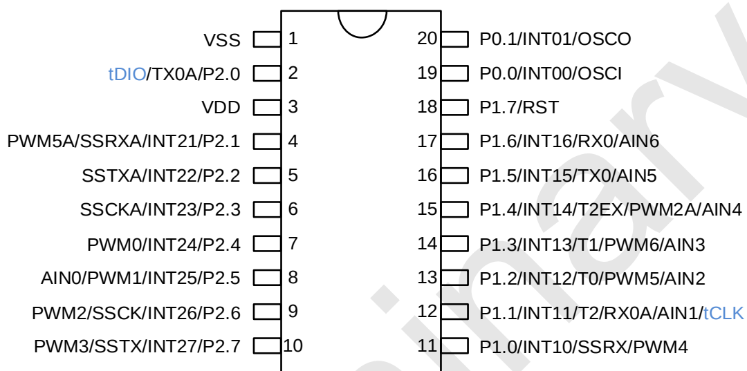
20PIN 管脚配置图
