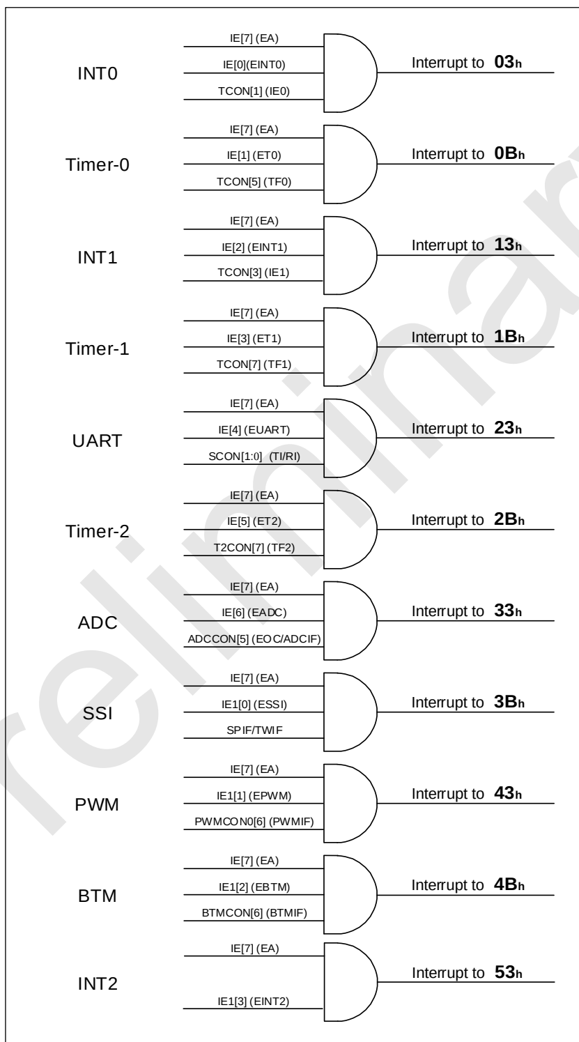
RD8G40x 中断结构和向量
