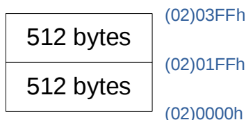
RD8G05 系列 EEPROM Sector 分区示意
