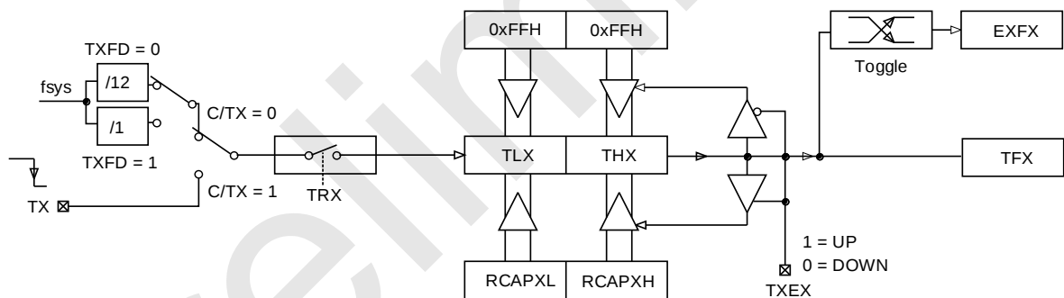
模式 1: 16 位自动重载 DCEN = 1
