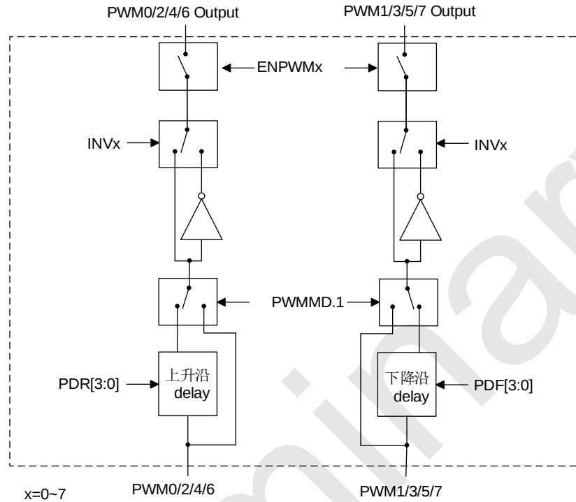
RD8G05 系列 PWM 互补模式框图
