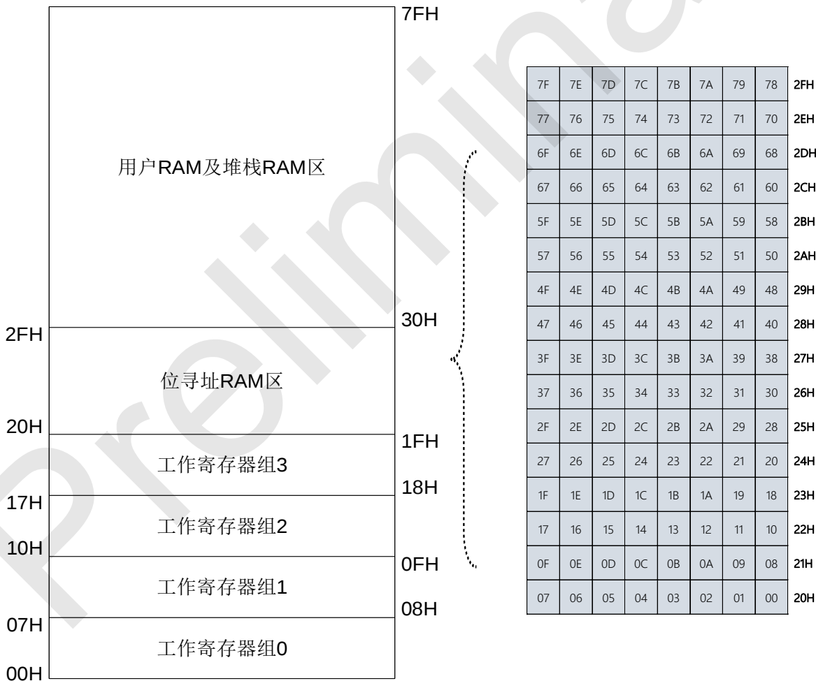
SRAM 结构图
