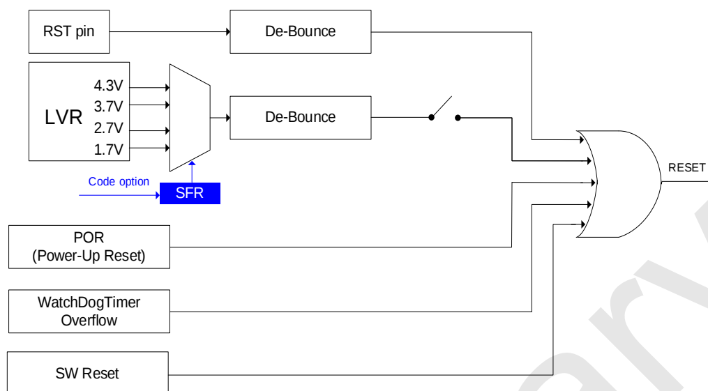
RD8G05 系列复位电路图
