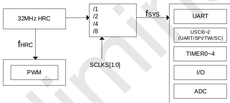
RD8G05 系列内部时钟关系
