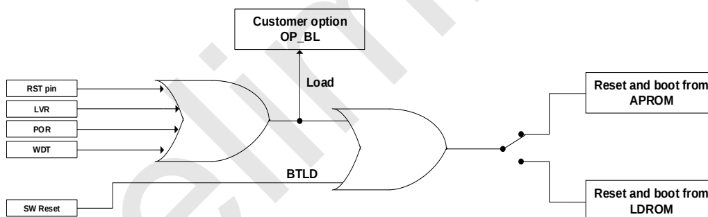
RD8G05 系列复位后启动区域切换示意图
