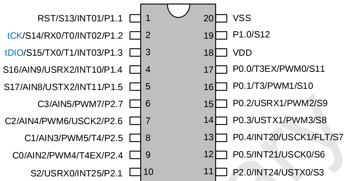
20PIN 管脚配置图
