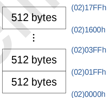
RD8G36 系列 EEPROM Sector 分区示意
