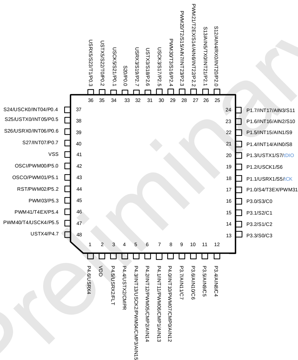
48PIN 管脚配置图
