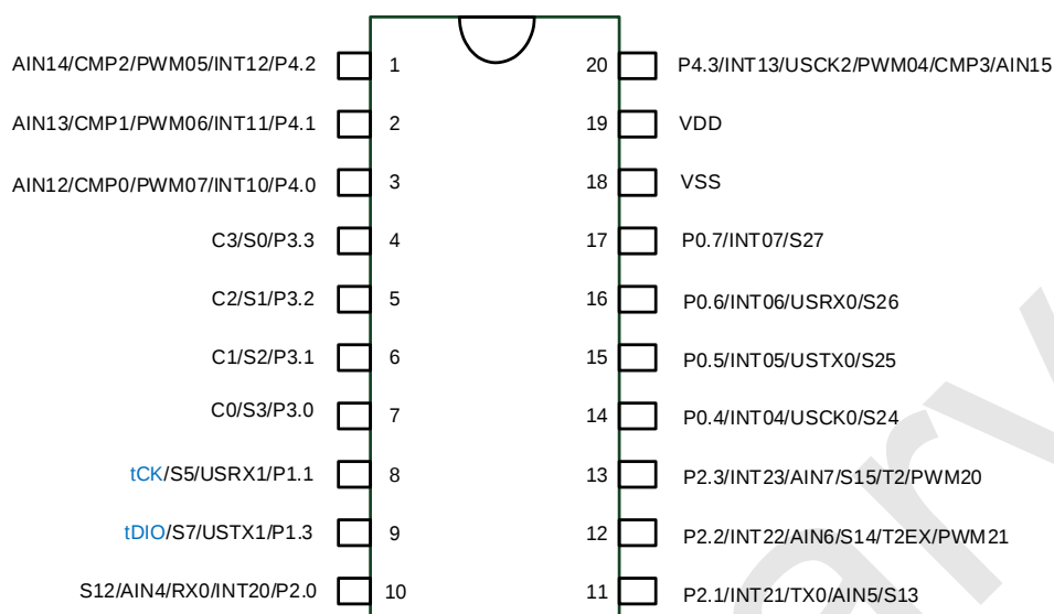
20PIN 管脚配置图
