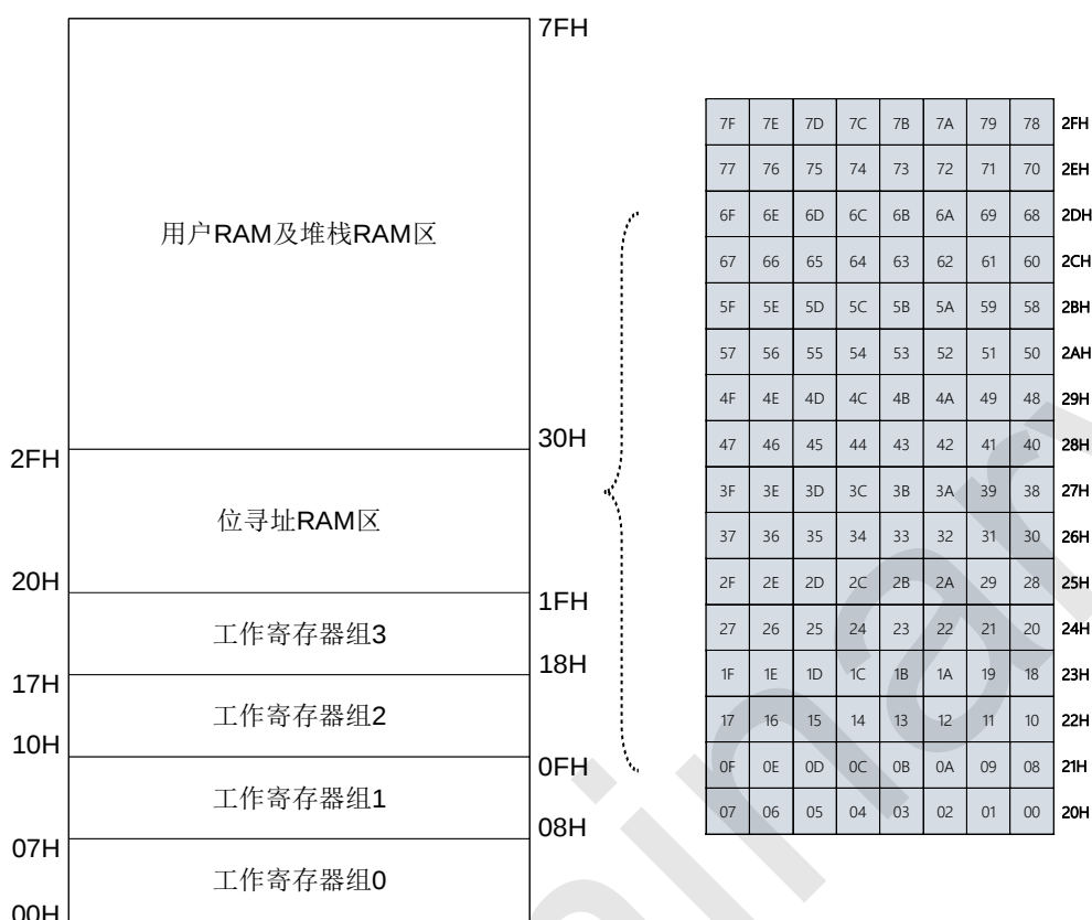
SRAM 结构图
