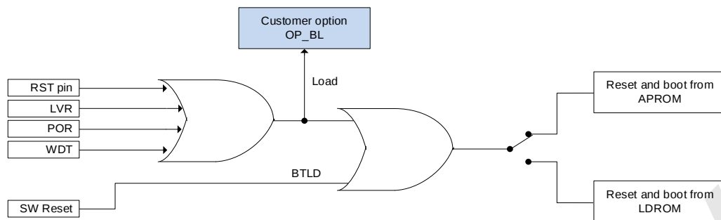
RD8G36 系列复位后启动区域切换示意图
