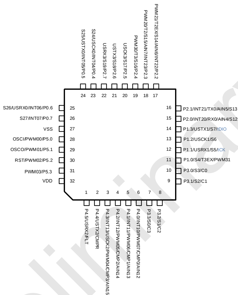
32PIN 管脚配置图
