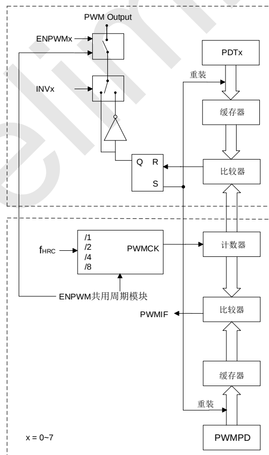
RD8G36 系列 PWM 结构框图
