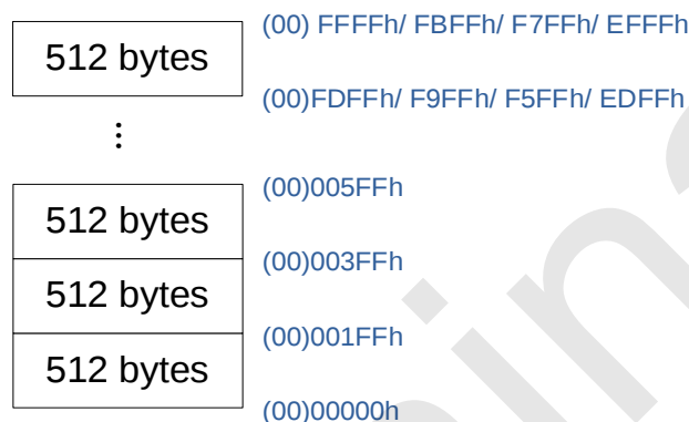
RD8G36 系列 64 Kbytes Flash ROM Sector 分区示意
