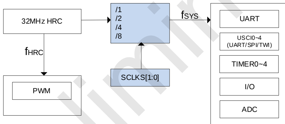
RD8G36 系列内部时钟关系
