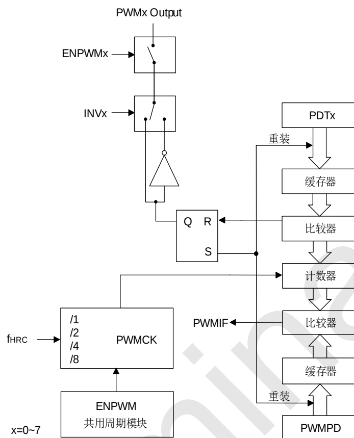
RD8G36 系列 PWM 独立模式框图
