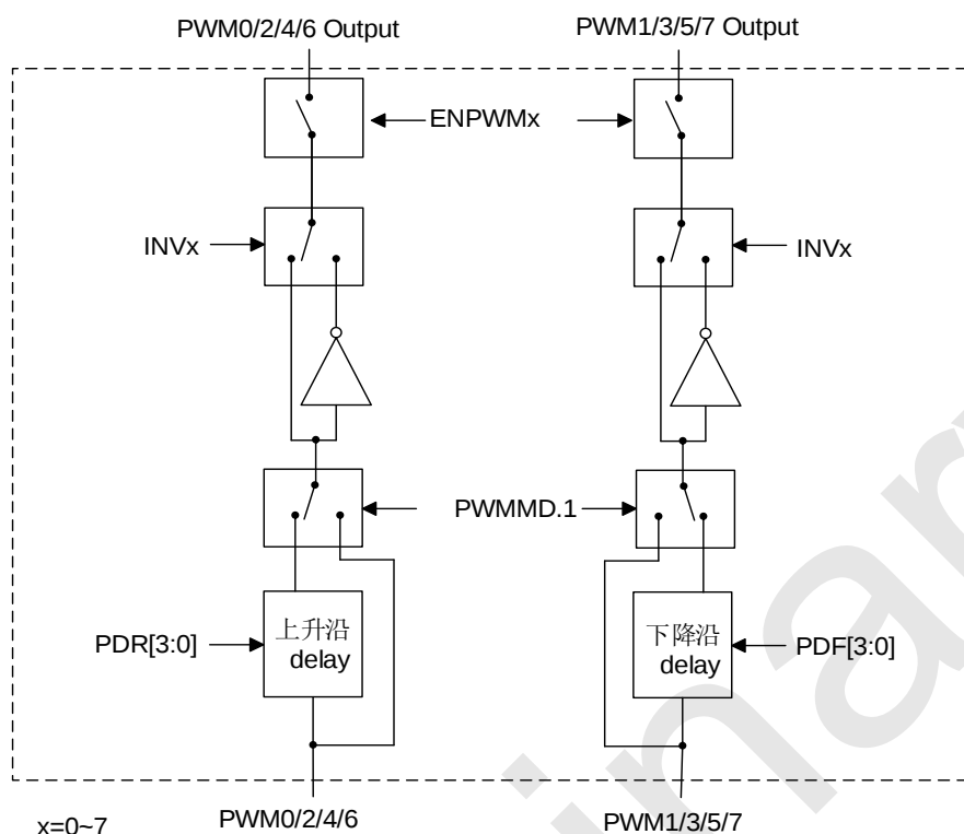
RD8G36 系列 PWM 互补模式框图
