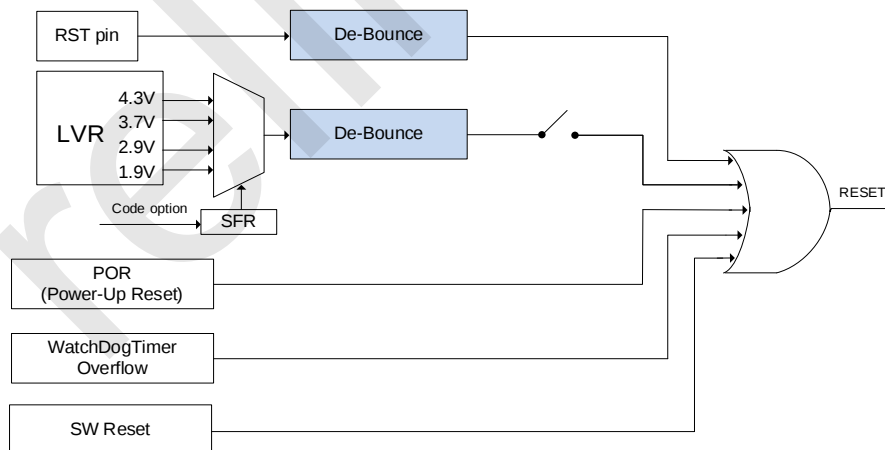
RD8G36 系列复位电路图
