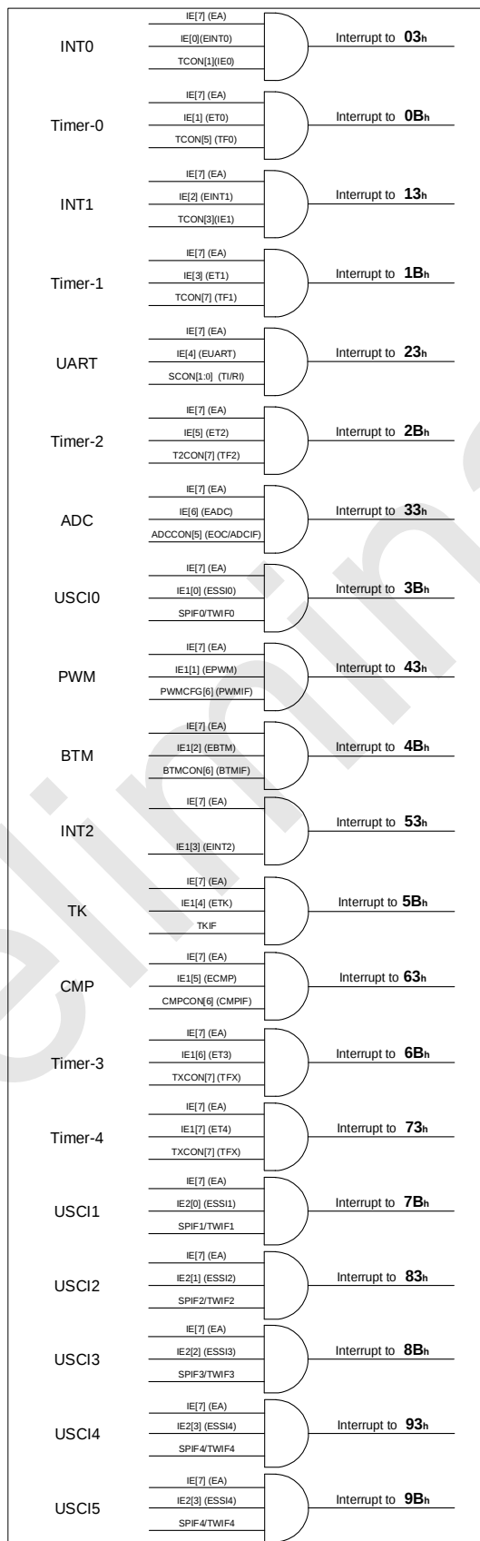
RD8G36 系列中断结构和向量
