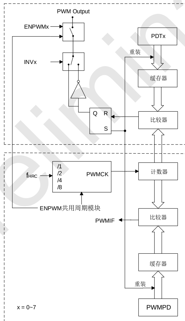
RD8T05 系列 PWM 结构框图
