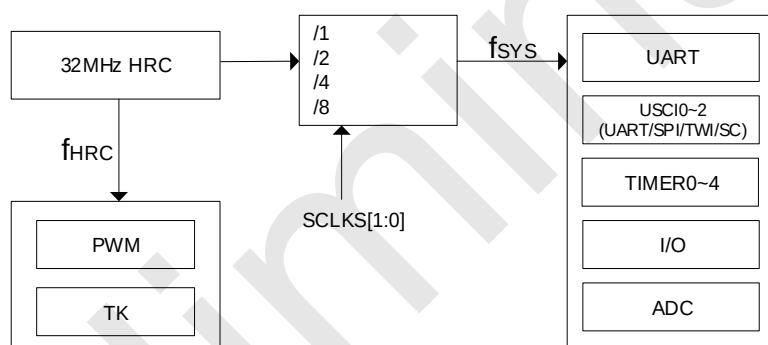
RD8T05 系列内部时钟关系
