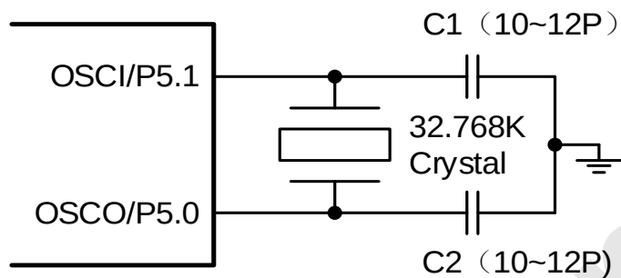
32.768kHz 外部晶振连接图
