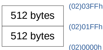
RD8T05 系列 EEPROM Sector 分区示意
