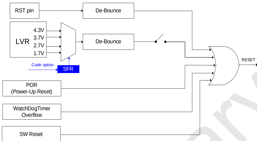
RD8T05 系列复位电路图
