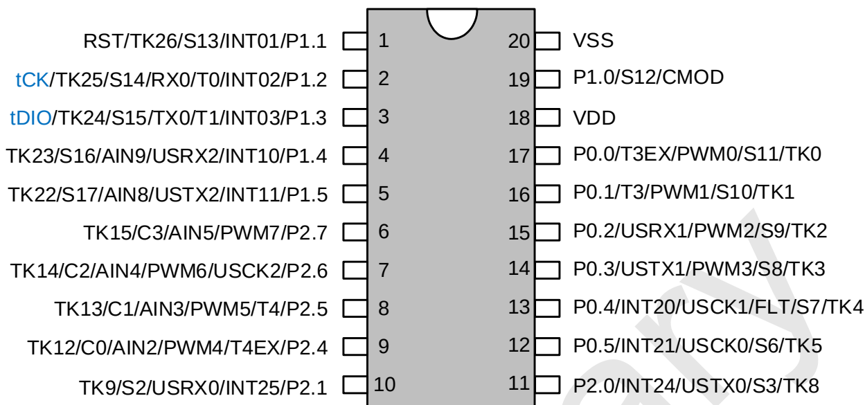
20PIN 管脚配置图
