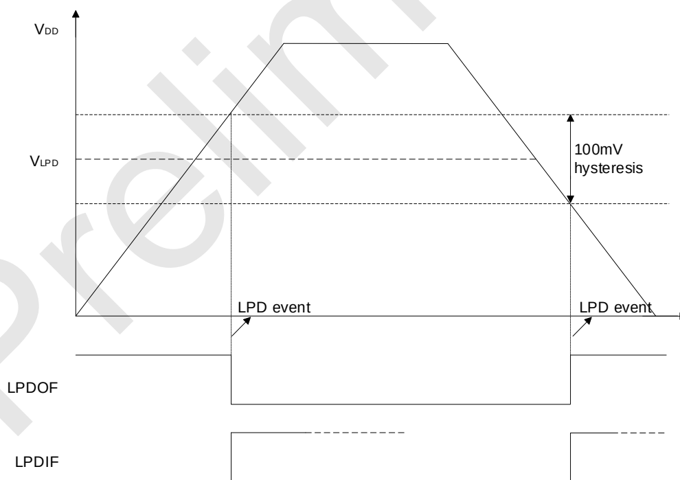
LPD 电压阈值
