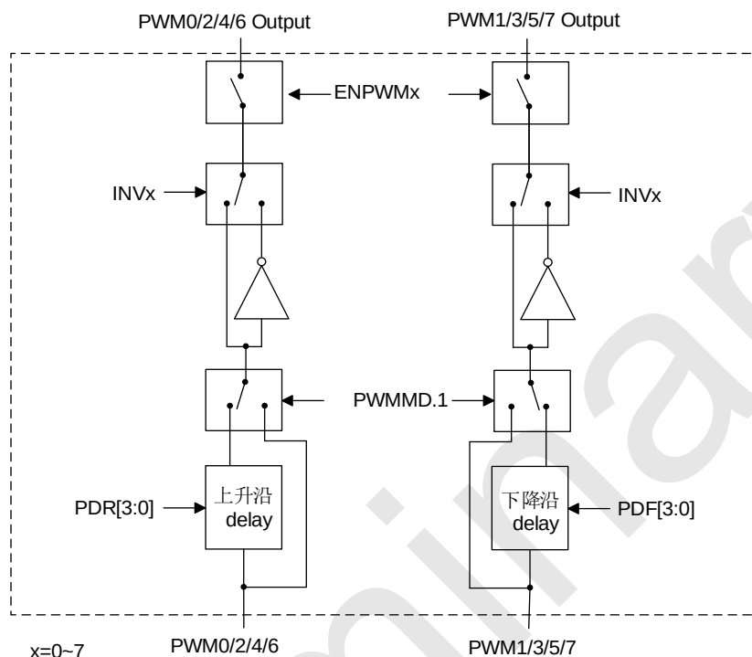
RD8T05 系列 PWM 互补模式框图
