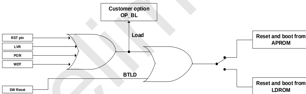
RD8T05 系列复位后启动区域切换示意图
