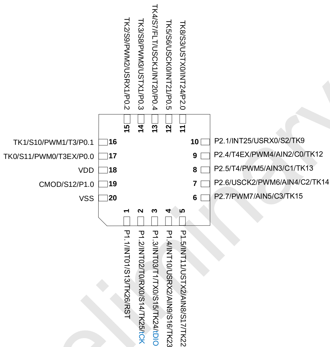
20PIN 管脚配置图
