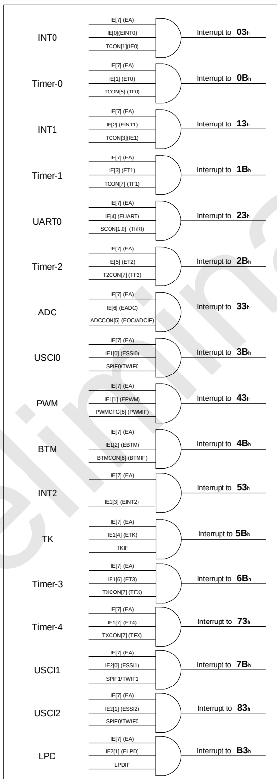
RD8T05 系列中断结构和向量
