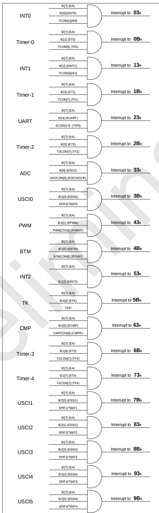
RD8T37 系列中断结构和向量
