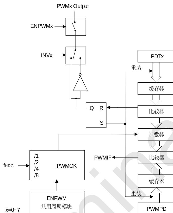
RD8T37 系列 PWM 独立模式框图
