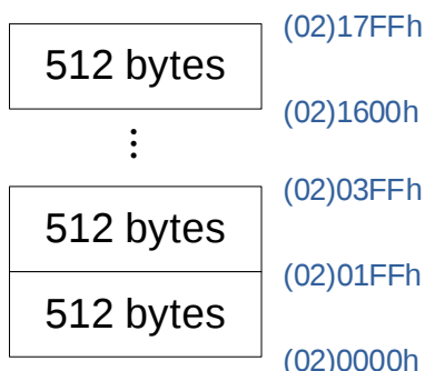
RD8T37 系列 EEPROM Sector 分区示意
