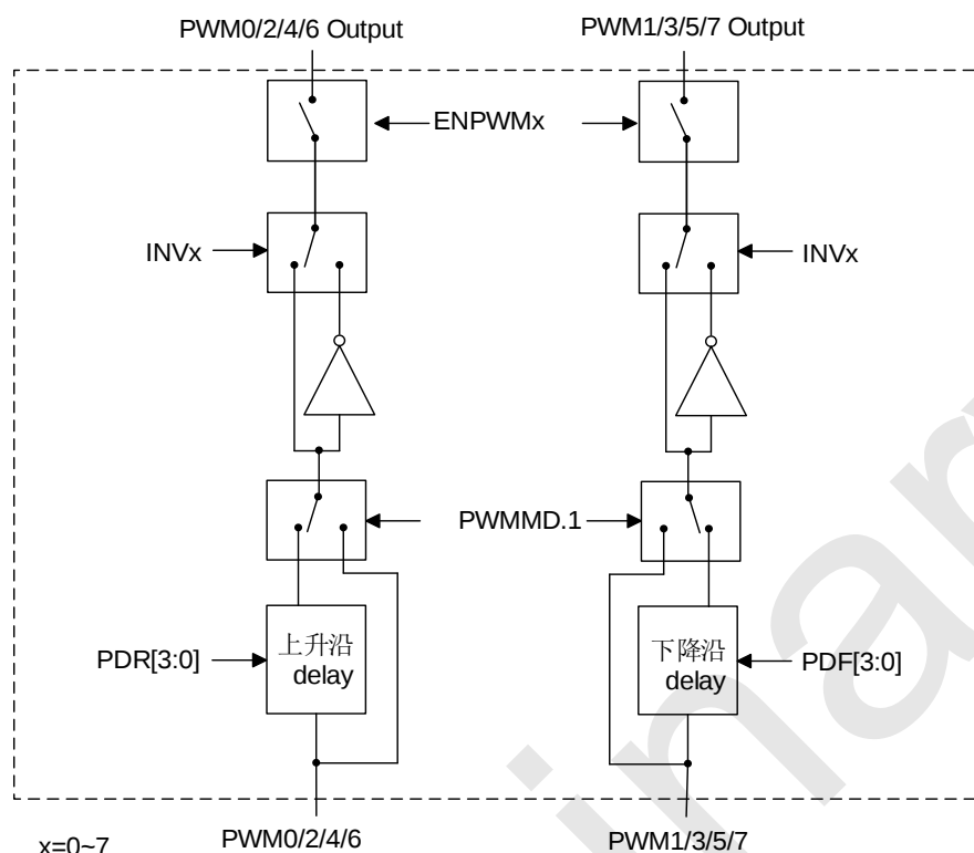
RD8T37 系列 PWM 互补模式框图
