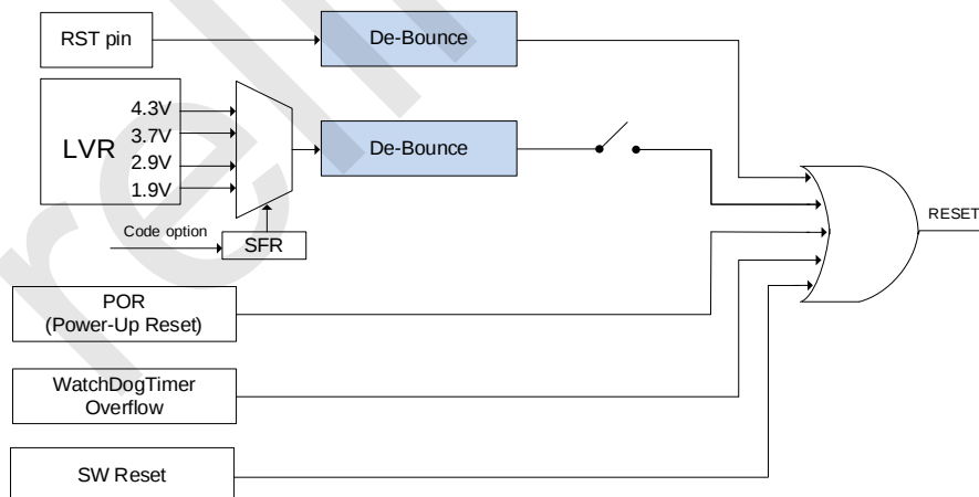
RD8T37 系列复位电路图
