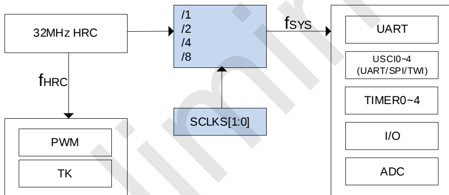
RD8T37 系列内部时钟关系
